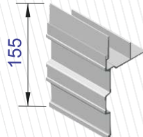
PERFIL SAIA 155mm SP COD: CR01003
