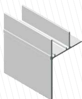
PERFIL SAIA 110mm SL
