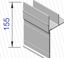
PERFIL SAIA 155mm SP COD: CR01004
